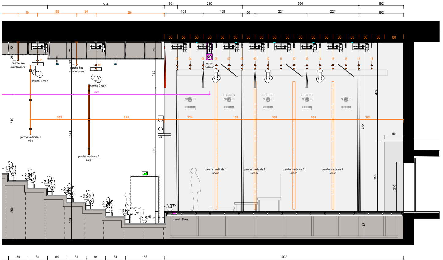
COUPE LONGITUDINALE SCENE
