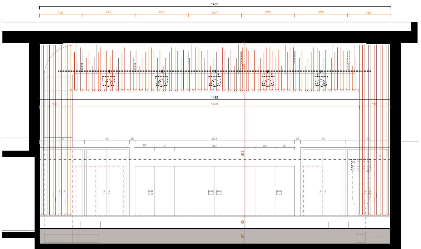
COUPE TRANSVERSALE SCENE
